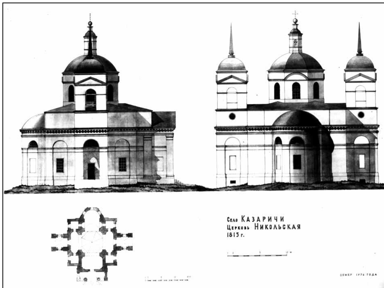
Рис. 5. Казаричи. Никольская церковь. Графическая реконструкция А.В. Прожеева (1977)
