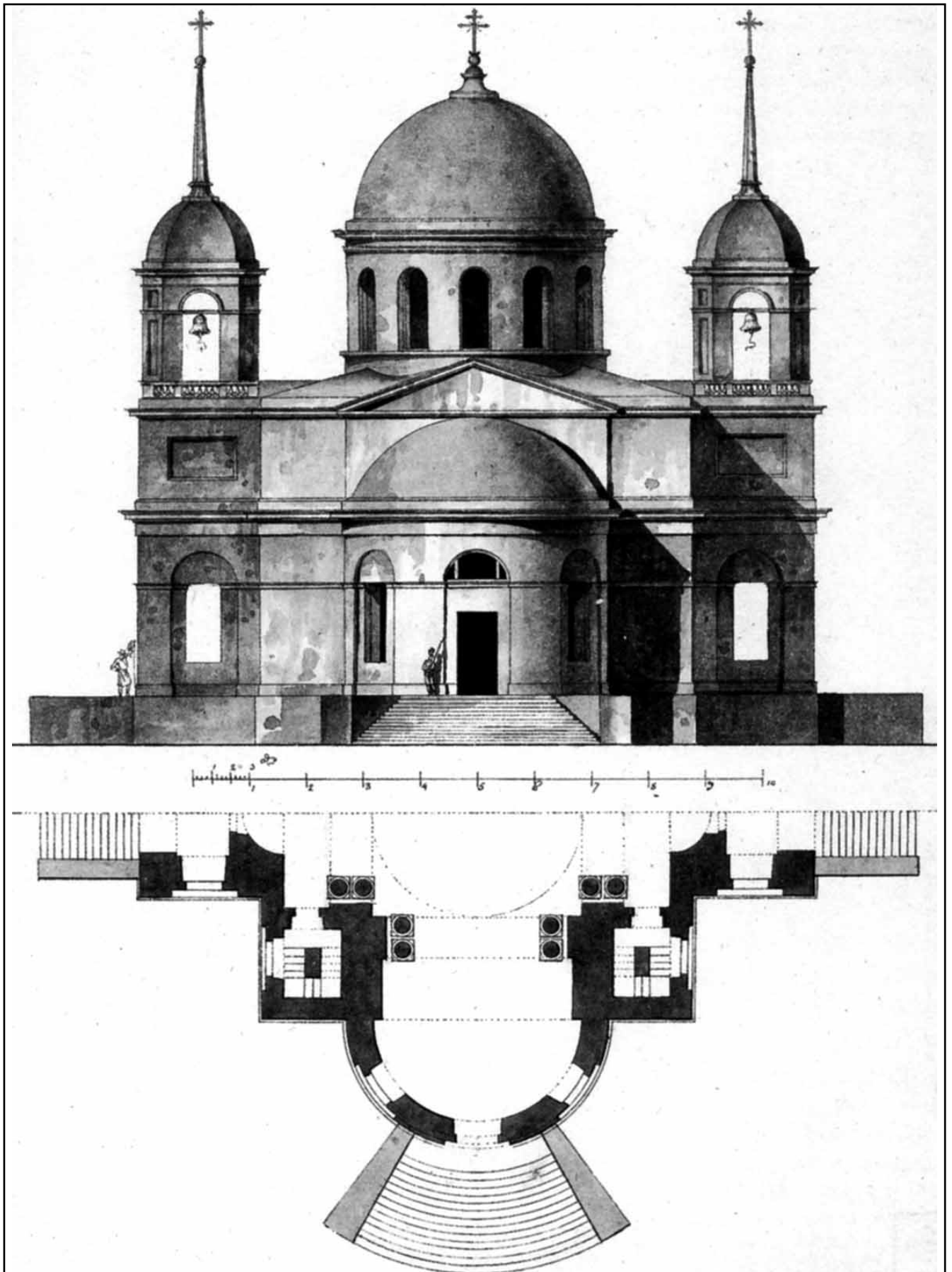
Рис. 4. Церковь Троицы в Дохновичах (Стародубский р-н, Брянской области). Авторский чертеж Н.А. Львова. Конец XVIII в.
