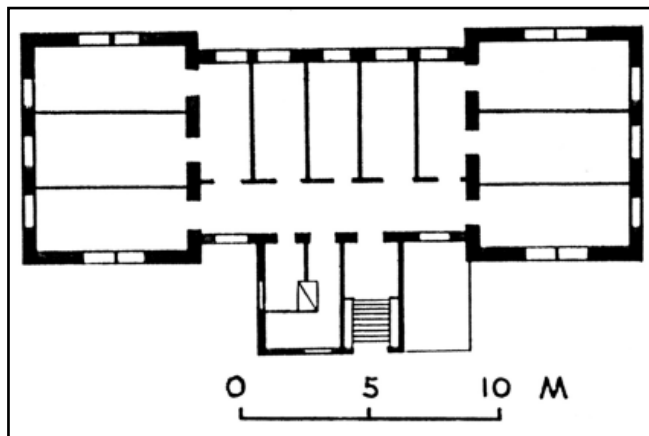
9. План першого поверху жіночого корпусу. Кресленник автора
