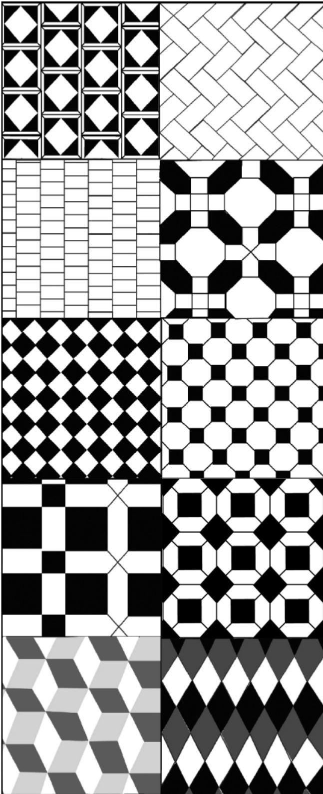
Рис. 14. Малюнок 10 конструкцій і орнаментів кам'яних і паркетних підлог, вживаних в спорудах Польщі на межі 17–18 ст., архітектора Тильмана ван Гамерена. Комп'ютерне редагування ілюстрації С. Дмитрієнка
