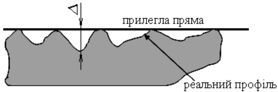
Рис. 1.15. Відхилення від прямолінійності
