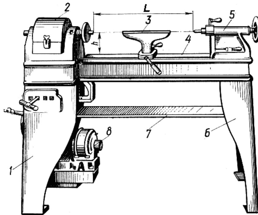
Рис. 1.32. Токарний верстат:
