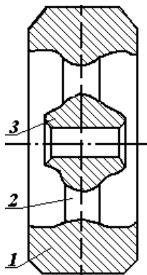
Рис. 2.12. Маховик
