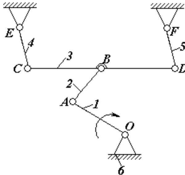
Рис. 2.4. Шарнірний механізм
