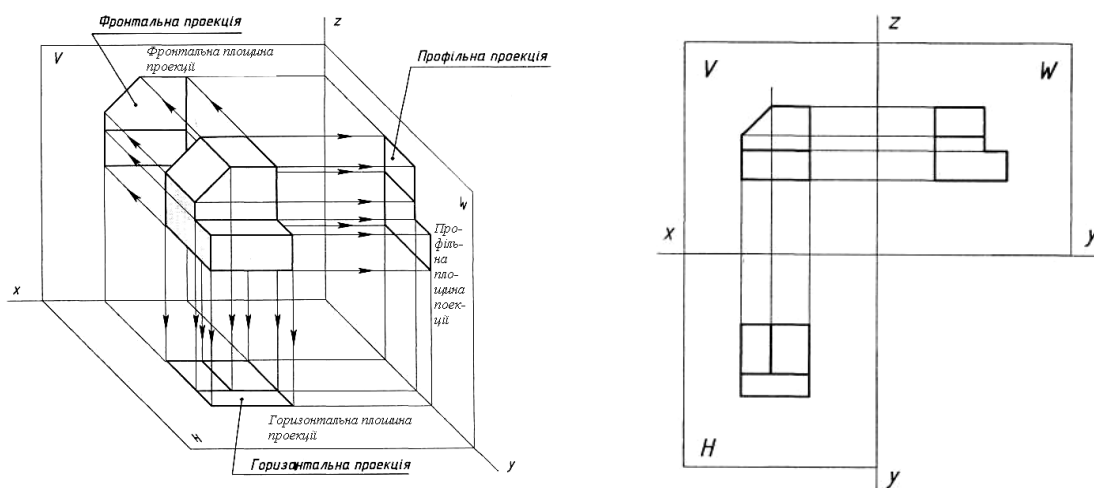
Рис. 1.43. Проєціювання предмета на три площини проєкцій
