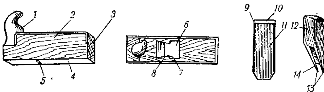
Рис. 3.10. Будова ручного рубанка: 1 – ріжок, 2 – колодка, 3 – затилоч, 4 – підшва, 5 – проліт, 6 – лоток, 7 – заплечики, 8 – щічки, 9 – фаска, 10 – лезо, 11 – ніж, 12 – клинок, 13 – вершини скосу, 14 – скіс
