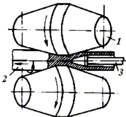
Рис. 1.4. Схематичне зображення косої прокатки: 1 – валики, 2 – заготовка, 3 – оправка.
