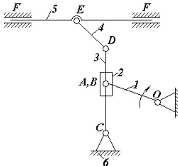
Рис. 2.3. Кулісний механізм
