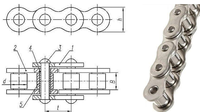
Рис. 2.34. Роликовий ланцюг
